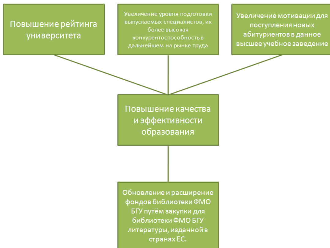
Рисунок 2. Дерево решений
